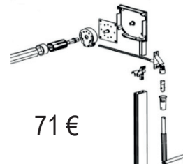
Acționare reductor cu manivelă pliabilă
