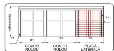
Rulouri cu casetă comună și plasă laterală
