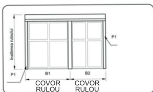
Rulouri cu casetă comună
